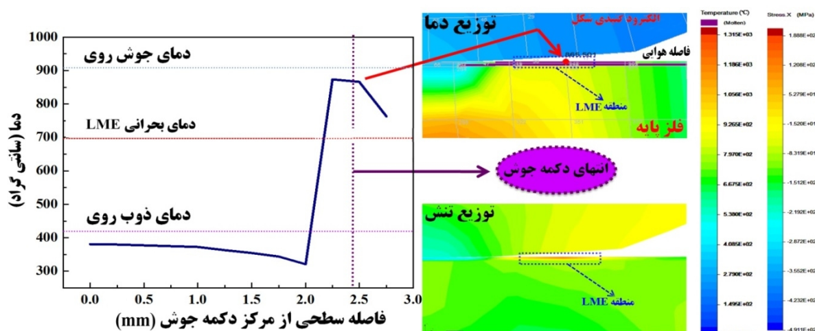
شکل 12- منحنی تغییر دمای سطح ورق مورد جوشکاری از مرکز (در تماس با مرکز الکترود) به سمت بیرون در انتهای سیکل جوشکاری و توزیع دما و تنش برای منطقه فوق بحرانی ترک‌دگی.
