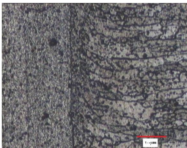
شکل ۳- ریزساختار مناطق اغتشاش و تحت تاثیر عملیات ترمومکانیکی
