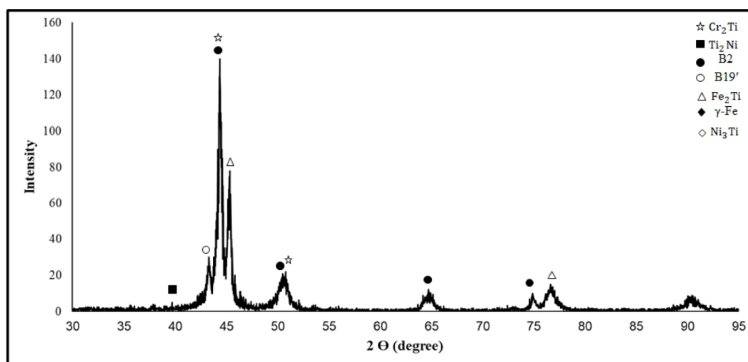
شکل 9- الگوی پراش پرتو ایکس منطقه جوش اتصال غیرهمجنس آلیاژ NiTi به فولاد زنگ نزن آستینیتی AISI 304.
