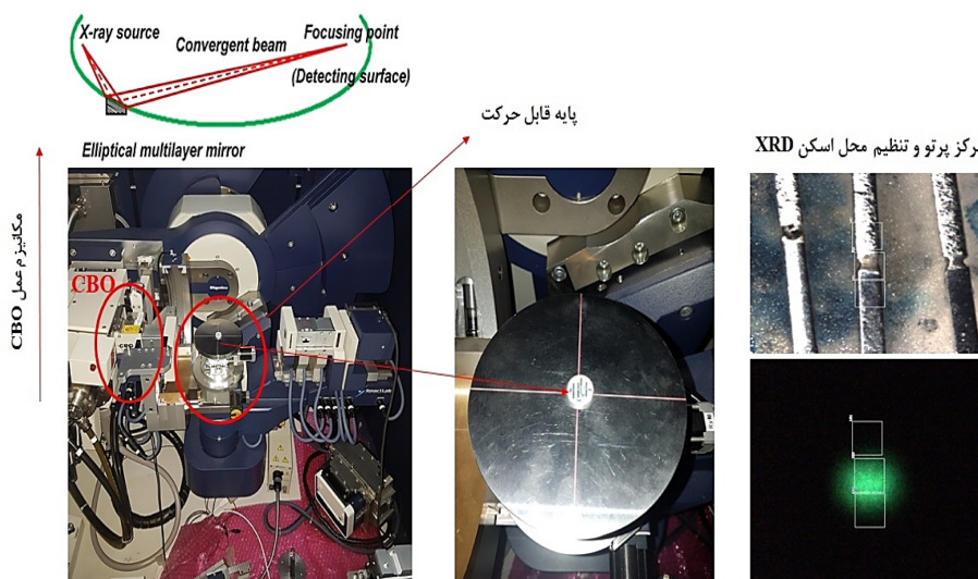
شکل 2- آزمون پراش پرتو ایکس در حالت متمرکز و مقیاس میکرو، دستگاه اسمارت لب شرکت ریگاکو [21].
