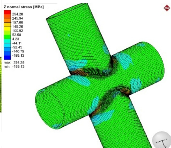
شکل ۱۹- توزیع تنش در راستای Z در اتصال جوشی
