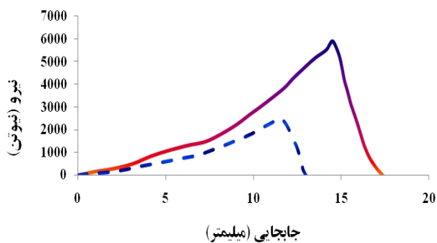
شکل ۴- نمودارهای نیرو - جابجایی جوش های نقطه ای مقاومتی با بیشترین و کمترین استحکام کششی - برشی
