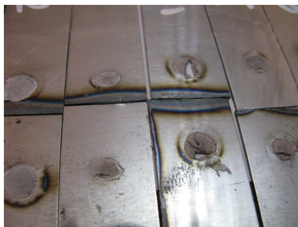
شکل ۳- جوش های نقطه ای مقاومتی پس از آزمایش کشش
