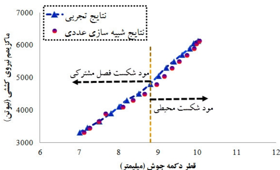
شکل ۱۳ - نتایج تجربی و شبیه سازی عددی تأثیر قطر دگمه جوش بر ماکزیم نیروی کششی جوشهای نقطه ای مقاومتی
