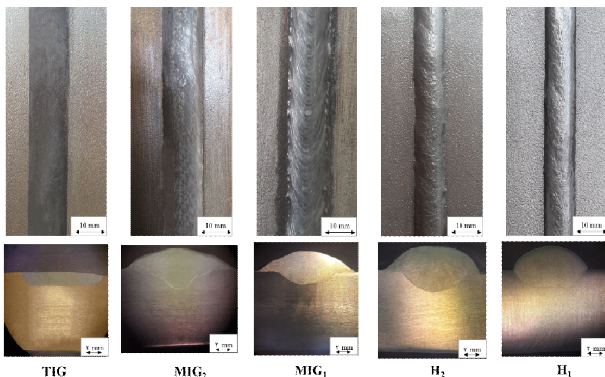
شکل ۷- شکل ماکرو از نمونه های جوش با شرایط ذکر شده در جدول ۴.
