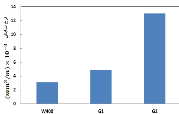
شکل 12- نرخ سایش برای سه نمونه.
