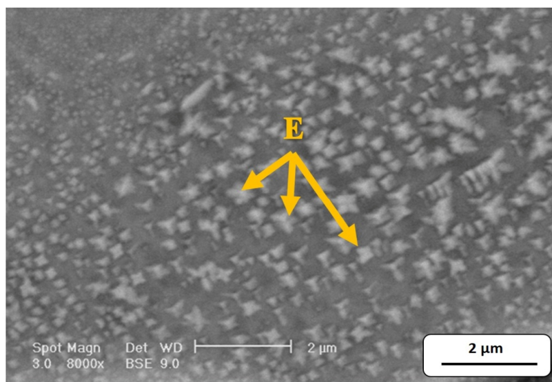
شکل ۷- تصویر میکروسکوپی الکترونی روبشی از فاز ستاره ای E در اطراف ناحیه انجماد غیرهمدمای
