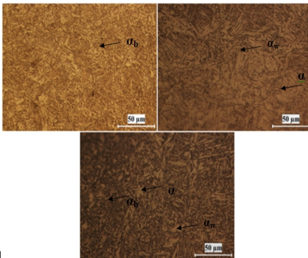
شکل ۴. منطقه اغتشاش یافته ناشی از جوشکاری اصطکاکی اغتشاشی فولاد X-60 (الف) FSW1000-60 (ب) FSW1000-60 (ج) 40 (ببیت = \alpha_b ، فریت = \alpha ، فریت ویدمن = \alpha_w )
