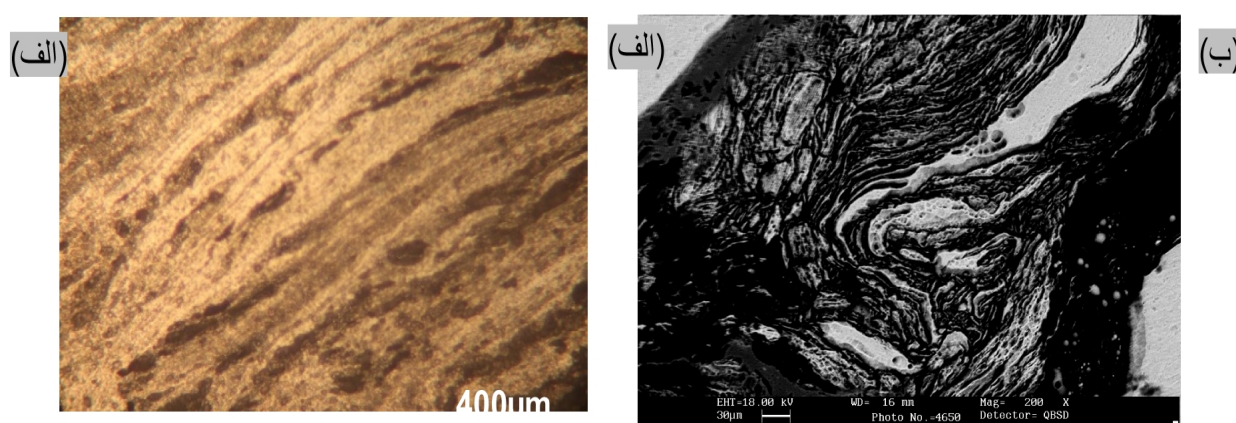
شکل ۶- (الف) تصویر میکروسکوپ نوری و (ب) تصویر میکروسکوپ الکترونی روبشی از ناحیه جوش
