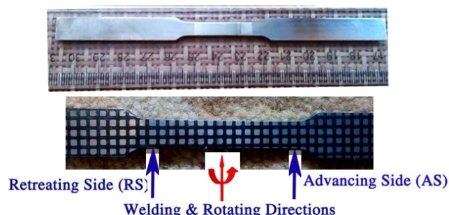
شکل ۱- نمونه کشش؛
