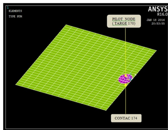
شکل 4- تماس پایلوت نود (target170) با ابزار.
