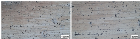
شکل 16- ریز ساختار فلز پایه در بزرگنمایی‌های مختلف.
