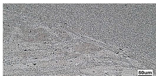
شکل 19- ریزساختار TMAZ در نمونه با شیار به عمق 1/5 میلی متر.
