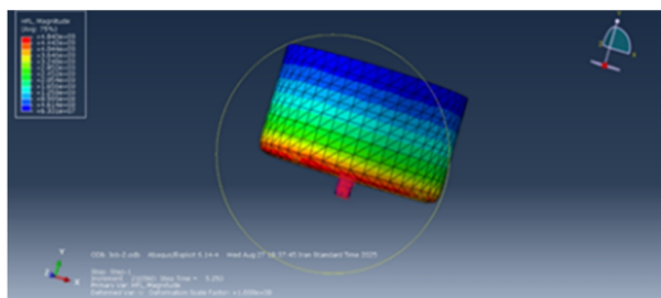
شکل 9- توزیع دما ابزار در پایان جوشکاری در سطح مقطع نمونه
