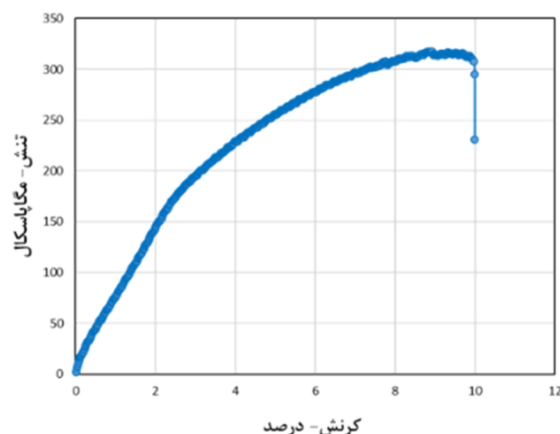
شکل 28- نمودار تنش کرنش نمونه 1/5 میلیمتر.
