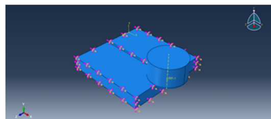
شکل 6- حرکت و بار در جهت ابزار داده شده در نرم افزار آباکوس.
