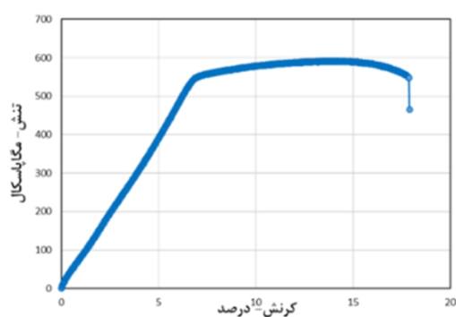
شکل 25- نمودار تنش کرنش رسم شده مهندسی از فلز پایه.
