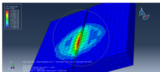
شکل 7- توزیع دما در پایان جوشکاری برای نمونه جوشکاری شده با عمق شیار 1/5 میلیمتری.
