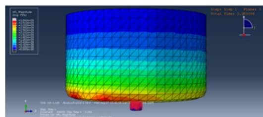
شکل 11- شیب دمایی در نمونه 1/5 میلیمتری در سرعت 1800 دور بر دقیقه.
