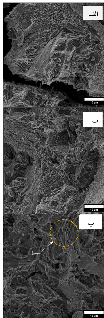
شکل 14- میکروسکوپ الکترونی در بزرگنمایی بیشتر، الف - نمونه A_1 ، ب - نمونه B1 و ج - نمونه B_2 .
