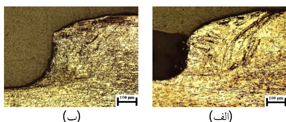
شکل 7- تصویر ماکروسکوپی کنار جوش نمونه با مدت زمان تماس 40 ثانیه و سرعت دورانی 1320 (الف)، 1800 (ب) و 2500 (پ)
