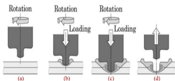
شکل 1- طرحواره فرایند جوشکاری اصطکاکی اغتشاشی نقطه ای (FSSW) [21].
