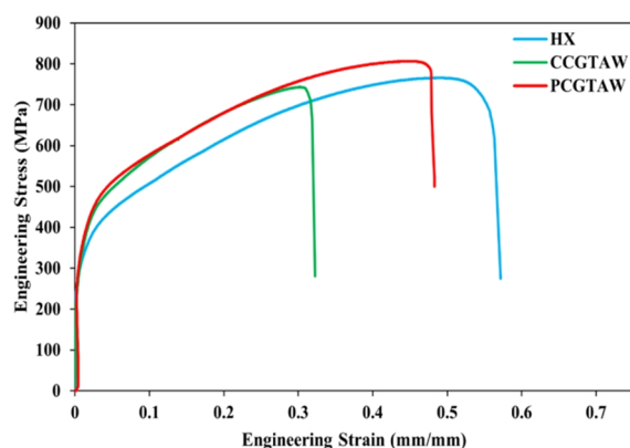
شکل 12- منحنی‌های تنش- کرنش فلز پایه و فلزهای جوش حاصل از فرایندهای مختلف
