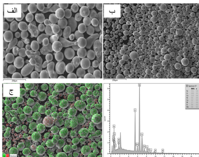
شکل 2- تصاویر SEM از سطح ذرات پودر الف - 17-4PH ب - Stellite6-17-4PH_{0.25} با آنالیز عنصری EDS.
