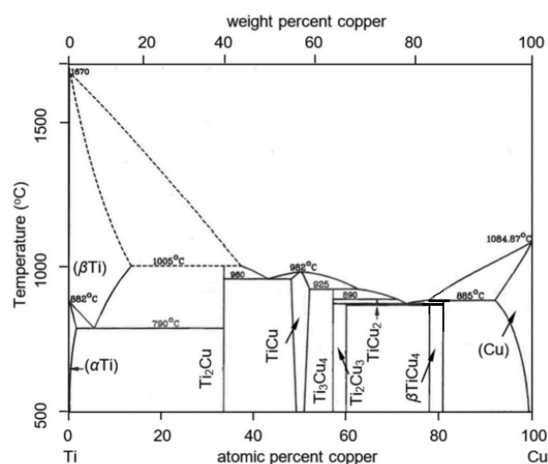
شکل 8- نمودار فازي Ti-Cu.
