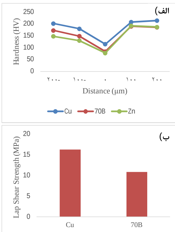
شکل 7- الف - داده‌های میکرو سختی سنجی فصل مشترک نمونه‌های دارای
