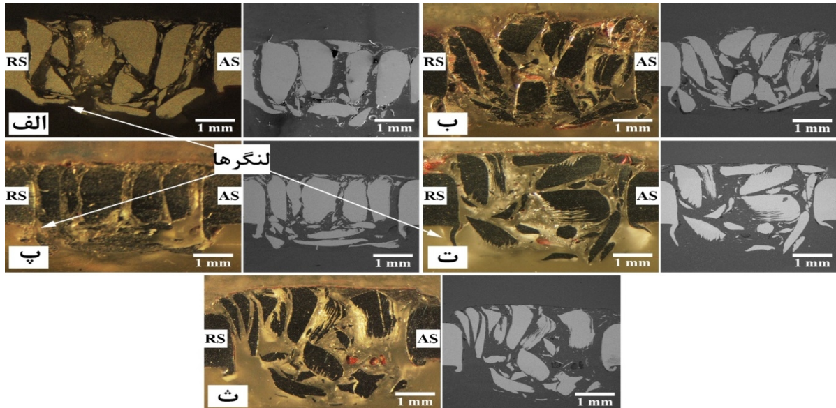
شکل 4- سطح مقطع اتصال و تغییر اندازه لنگرها در نمونه‌های جوشکاری شده با سرعت چرخشی در نمونه‌های
