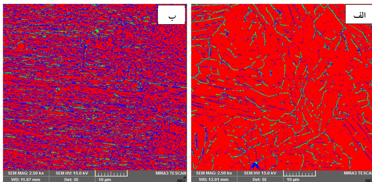
شکل 4- توزیع فازهای فریت و آستنیت در ریزساختار فلزجوش فولاد 17-4PH: الف - شرایط as-weld و ب - شرایط فرایپرسیازی دو مرحله‌ای.
