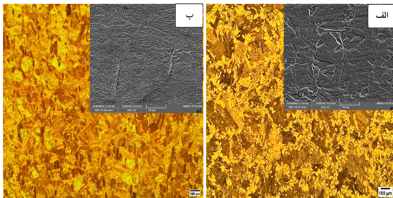
شکل 2- ریزساختار ناحیه HAZ فولاد 17-4PH در شرایط: الف - as-weld و ب- فرایپرسیازی دو مرحله ای.
