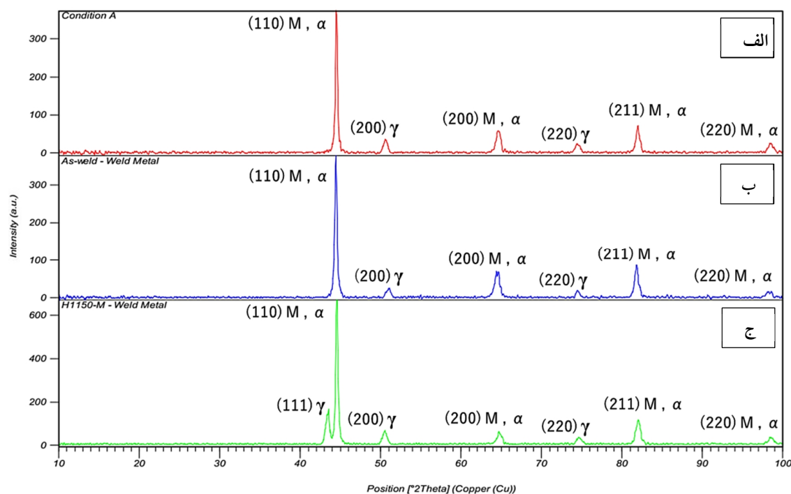
شکل 5- پروفیل های XRD: الف - نمونه آنیل انحلالی ب- فلزجوش در شرایط as-weld ج- فلزجوش در شرایط فرایپیرسازی دو مرحله‌ای.
