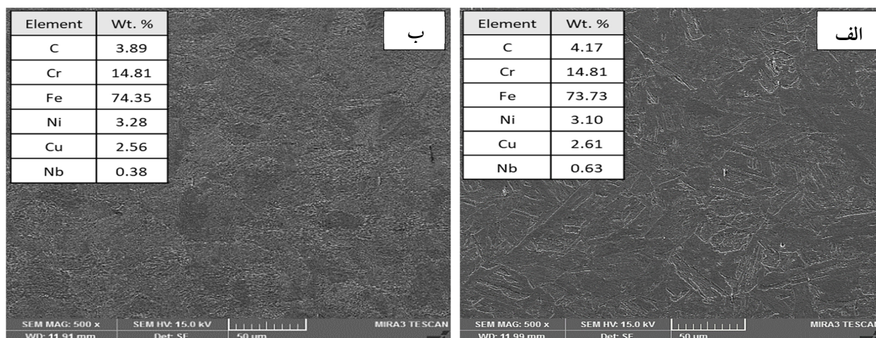
شکل 6- تصویر میکروسکوپ الکترونی به همراه آنالیز EDS فلز پایه فولاد 17-4PH الف- در حالت آنیل انحلالی ب- در حالت فرایپرسی دو مرحله‌ای.
