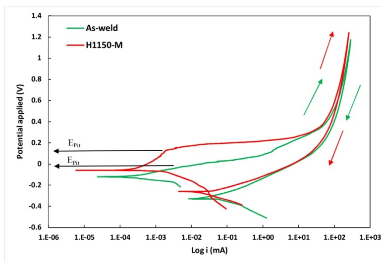
شکل 8- نمودار مقایسه ای پلاریزاسیون چرخه‌ای فلزجوش فولاد 17-4PH در دو شرایط as-weld و فرایپیرسازی دو مرحله ای
