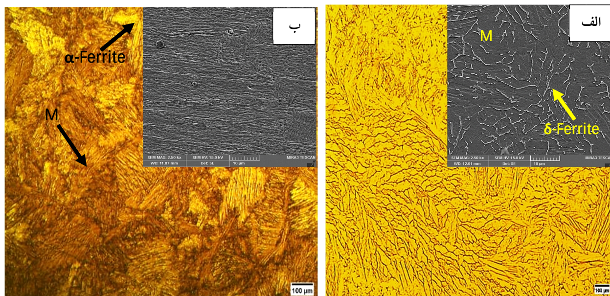
شکل 3- ریزساختار فلزجوش فولاد 17-4PH در شرایط: الف - as-weld و ب - فرایپرسیازی دومرحله‌ای
