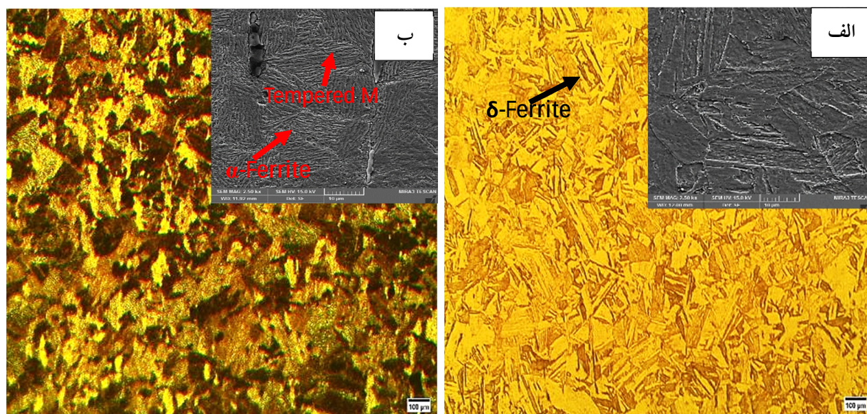
شکل 1- ریزساختار فلز پایه فولاد 17-4PH در شرایط: الف - آنیل انحاللی و ب- فرایپرسیازی دو مرحله ای
