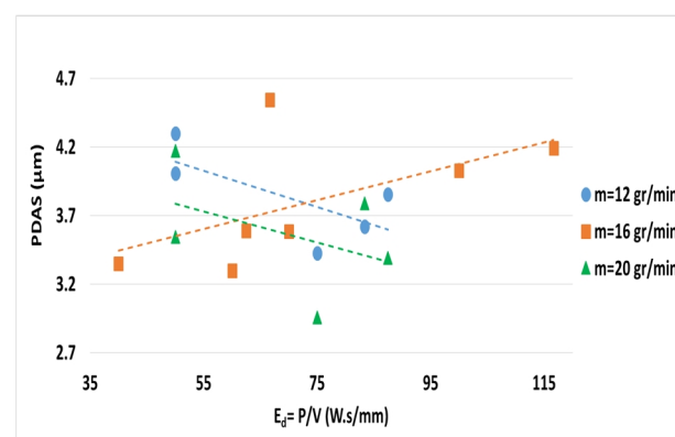
شکل 8- ابعاد بازوهای دندردیتی اولیه برحسب چگالی انرژی در نرخهای پاشش پودر مختلف.
