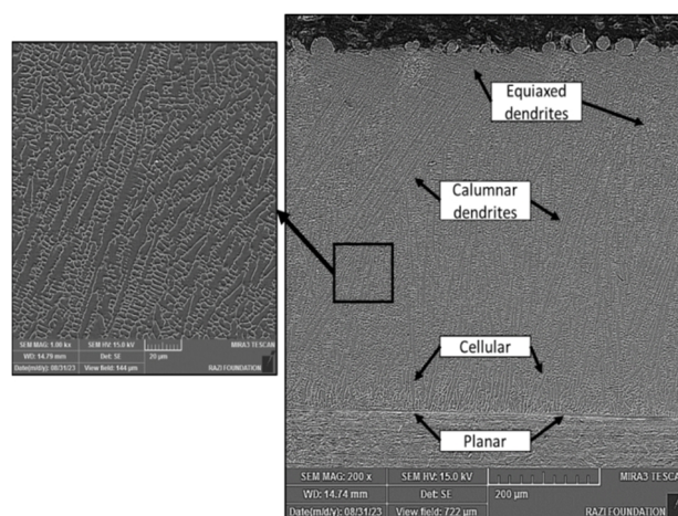
شکل 7- تصویر میکروسکوپی الکترونی روبشی سطح مقطع طولی نمونه تک‌پاس، رشد دندردیت‌های ستونی در جهت خلاف انتقال (اتلاف) حرارت.
