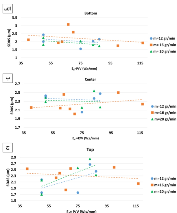
شکل 9- ابعاد بازوهای دندردیتی ثانویه برحسب چگالی انرژی در نواحی الف - پایینی، ب - میانه و ج - مرکز و بالای روکش ایجادشده در نرخهای پاشش پودر مختلف.
