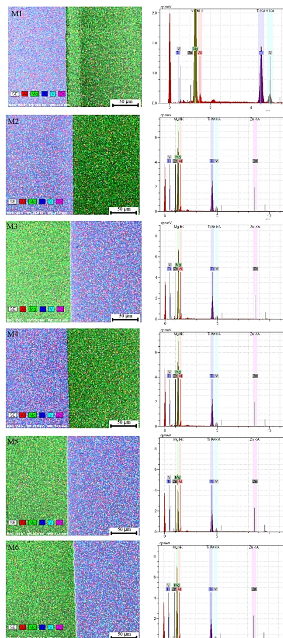
شکل 4- آنالیز نقشه EDS و نمودار فراوانی عناصر از سطح مقطع منطقه اتصال (سمن) AZ31 تا M6.
