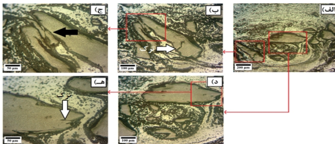
شکل 7- تصویر میکروسکوپی نوری ریزساختار منطقه کامپوزیتی نمونه جوشکاری شده با سرعت چرخش 250 دور در دقیقه و سرعت پیشروی 20 میلی متر بر دقیقه الف- قسمتی از منطقه اغتشاشی، ب-ه- تصاویر متناظر با بزرگمایی بالاتر.
