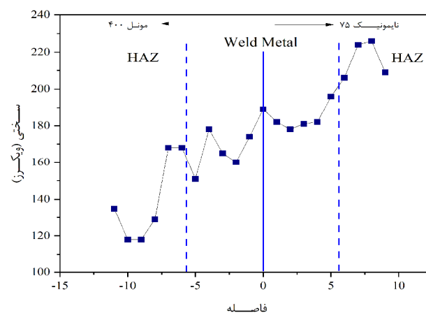
شکل 5- نمایه ریز سختی در مقطع جوش نمونه شماره 11. xzs.
