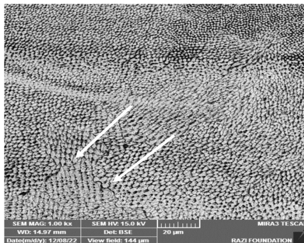
شکل 2- رسوبات مختلف تشکیل شده در نواحی ریزساختار جوش نمونه
