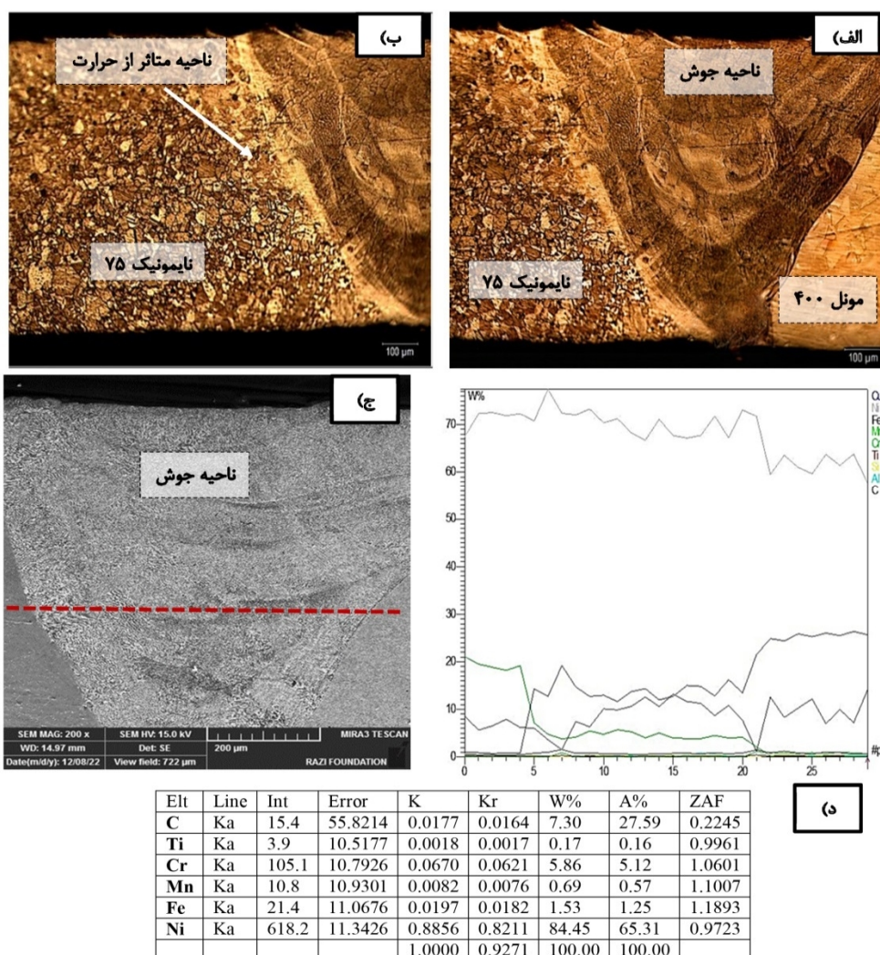
شکل 1- الف و ب- تصویر میکروسکوپ نوری از ناحیه جوش نمونه شماره 11
