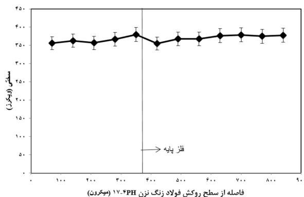
شکل 14- تغییرات ریزسختی پوشش فولاد زنگ نزن 4PH-17 و زیرلایه برحسب فاصله از سطح پوشش.
