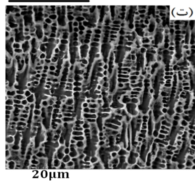
شکل 4- تصویر میکروسکپی الکترونی روبشی از ریزساختار مقطع عرضی
