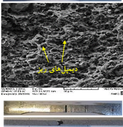
شکل 10- تصاویر SEM از گشش شکست نمونه های الف- RS ب- As-Weld ج- AS.
