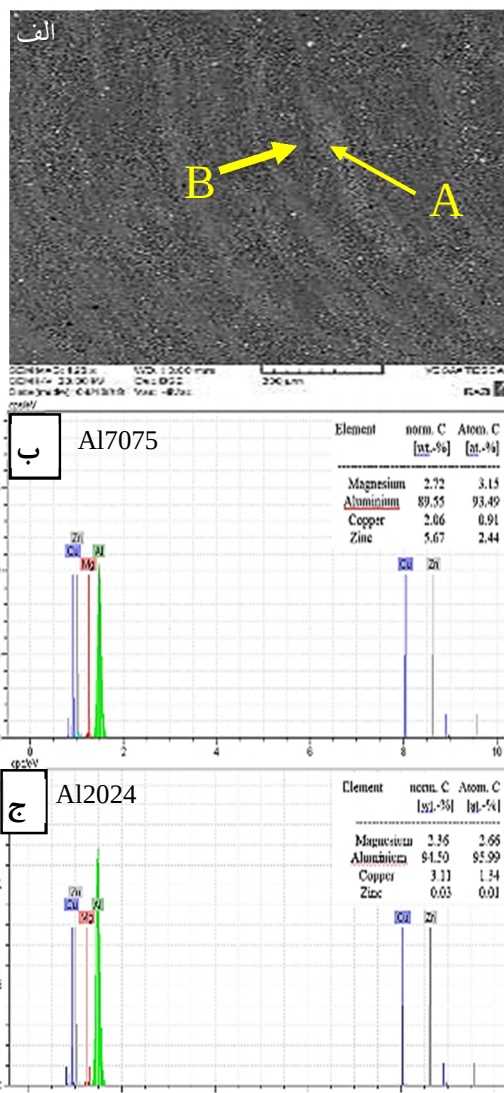
شکل 7- الف - تصویر SEM از ناحیه اغتشاش یافته از نمونه AS و آنالیز EDS از ب - نقطه A ج - نقطه B
