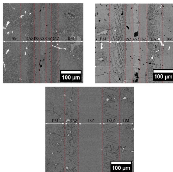
شکل 2- تصویر میکروسکپ الکترونی روبشی از محل اتصال نمونه‌های متصل شده در دمای الف - 1060°C، ب - 1120°C، ج - 1180°C و زمان 45 دقیقه.
