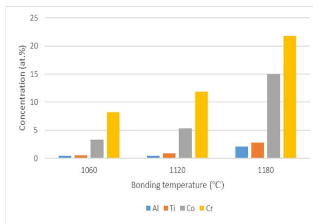
شکل 4- میانگین غلظت چهار عنصر Al, Ti, Co, Cr در ناحیه ISZ نمونه‌های متصل شده در دماهای 1060°C، 1120°C و 1180°C.
