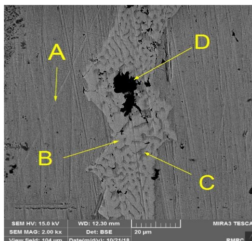
شکل 8 - تصویر میکروسکوپ الکترونی روبشی از محل اتصال نمونه متصل شده در دمای 1120°C و زمان 45 دقیقه. فازهای A, B, C و D در تصویر مشخص هستند که به ترتیب فازهای پرویوتکتیک- \gamma ، بورید غنی از نیکل، یوتکتیک- \gamma و بورید غنی از کروم هستند.
