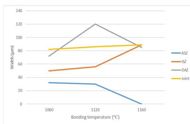
شکل 5- اثر دمای اتصال بر ضخامت نواحی ASZ، ISZ و DAZ و کل ناحیه اتصال.
