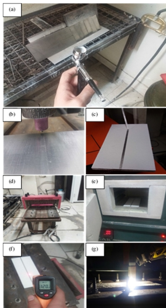
شکل 3- مراحل آماده‌سازی و اعمال جوشکاری به روش (FB-TIG, a نحوه قرار دادن نمونه اصلی و نمونه‌های شاهد در کنار هم جهت پاشش فلاکس، (b) جانمایی نمونه در محل جوش قبل از پاشش فلاکس (c) جدا کردن چسب از روی نمونه بعد از پاشش فلاکس جهت ایجاد شیار بین فلاکسی، (d) گرم کردن میز جوشکاری، (e) پیش گرمایش نمونه‌های S4 تا S9 در کوره، (f) کنترل دما توسط دماسنج لیزری برای تعیین زمان شروع جوشکاری، (g) نمایی از جوشکاری نمونه‌ها
