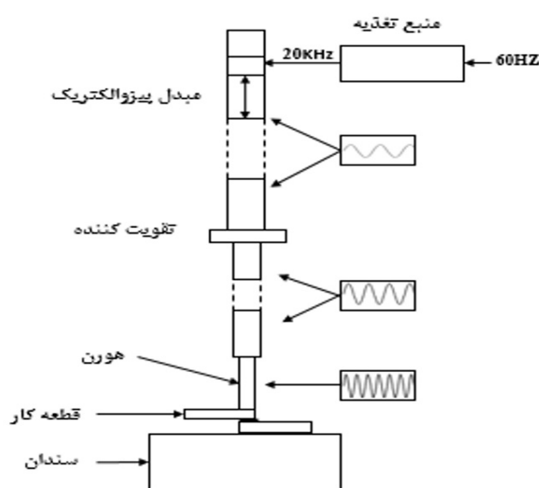
شکل 1- شمای دستگاه جوشکاری فراصوتی.
