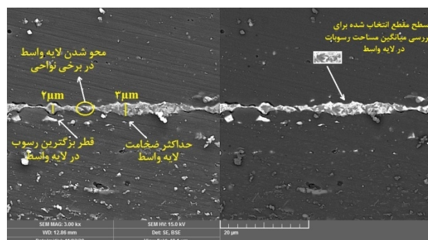
شکل 10- تصویر میکروسکوپ الکترونی از محل اتصال با ضخامت لایه واسط 20 میکرومتر پس از 210 دقیقه ماندگاری در کوره.
