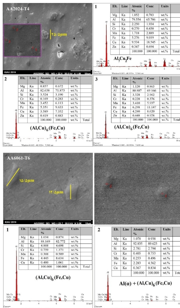
شکل 1- تصویر میکروسکوپ الکترونی فلزات پایه پیش از اعمال فرایند فاز مایع گدا.
