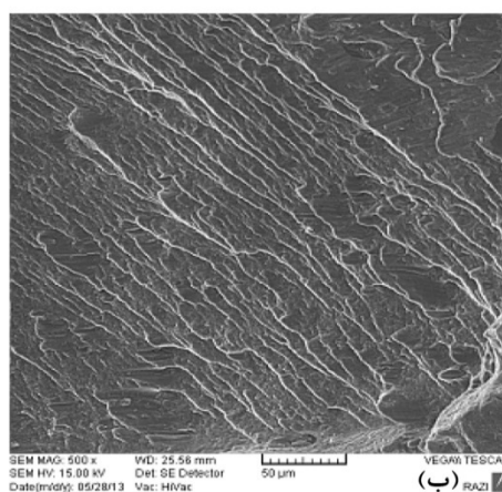
شکل 14- ماکروگراف SEM سطح شکست نمونه خستگی آلیاژ آلومینیوم ریختگی فرآوری شده FSP تحت تنش اعمالی 170MPa (الف) حضور علائم چرخ‌دنده‌ای (منطقه رشد ترک) در موقعیت‌های ساعت 4 و 10، (ب) حضور خطوط توقفی مرتبط با دوره‌های رشد ترک و (ج) انحراف مسیر رشد ترک در ناحیه بارگذاری زیاد.
