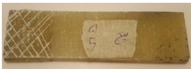
شکل 4- یک نمونه آماده شده جهت جوشکاری فراصوتی
