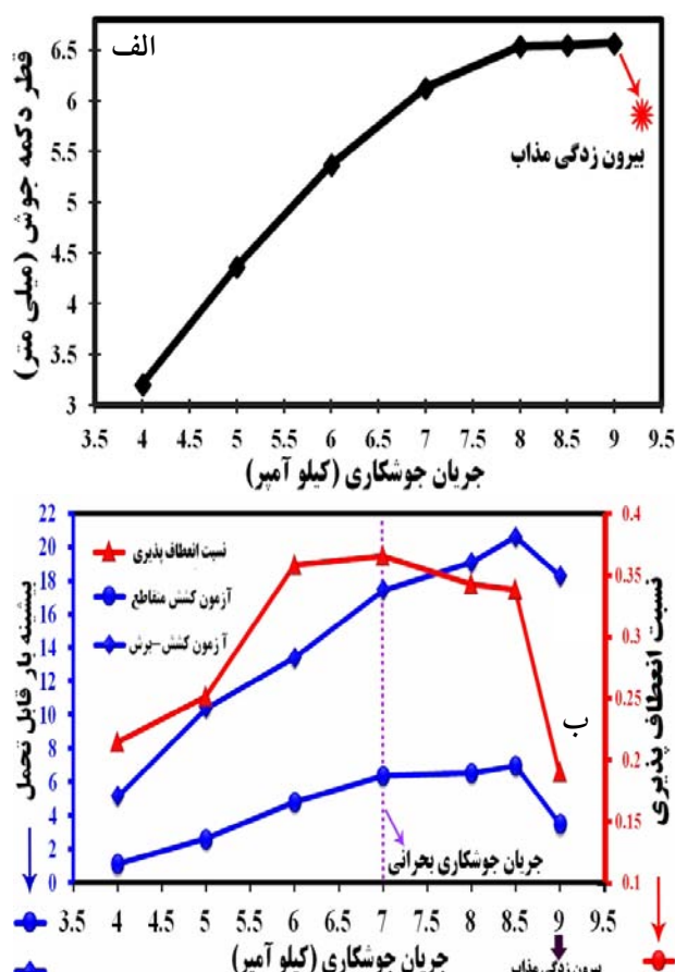
شکل 3- تغییر الف) اندازه دکمه جوش و ب) حداکثر بار قابل تحمل در آزمون کشش-برش (TSS) و حداکثر بار قابل تحمل در آزمون کشش متقاطع (CTS) فولاد TRIP با جریان جوشکاری.
