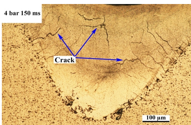
شکل 13- سطح مقطع نمونه 4P150، ترک‌ها نسبت به نمونه 4P20 کمتر هستند.
