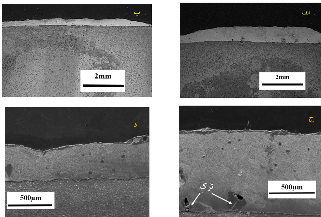
شکل 4- تصویر میکروسکوپی الکترونی روبشی: الف) و ج) هم پوشانی تک پاس های روکش 75 درصد، ب) و د) هم پوشانی تک پاس های روکش 50 درصد
