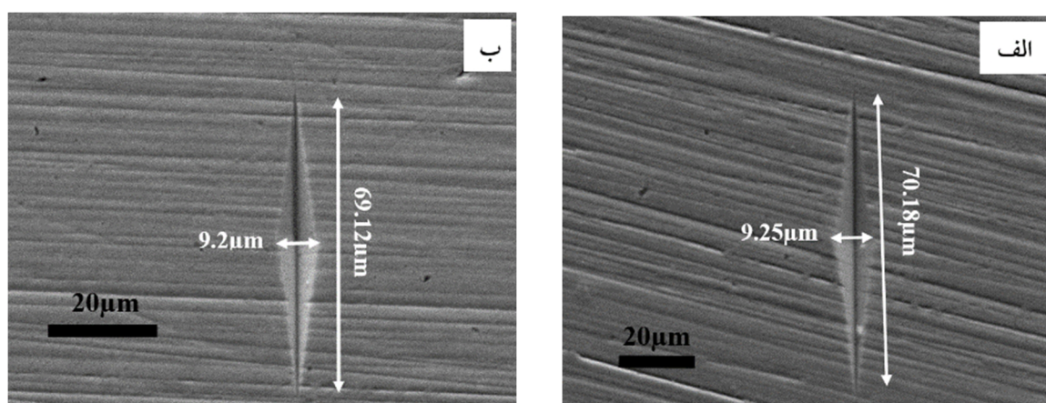
شکل 8- تصاویر میکروسکوپی الکترونی از اثر دندانه گذاری فرورونده ویکرز روی سطح مقطع پوشش:
