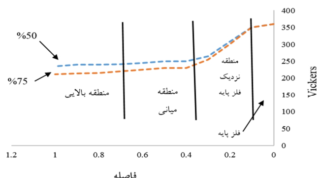
شکل 7- نمودار ریزسختی پوشش با هم پوشانی تک پاس های روکش 50 و 75 درصد
