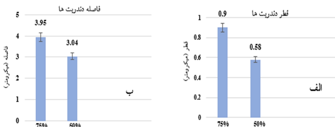
شکل 6- الف) نمودار ضخامت ستون های دندردیت ها نزدیک سطح پوشش در هم پوشانی تک پاس های روکش 75 و 50 درصد و ب) نمودار فاصله دندردیت ها نزدیک سطح پوشش در هم پوشانی تک پاس های روکش 75 و 50 درصد
