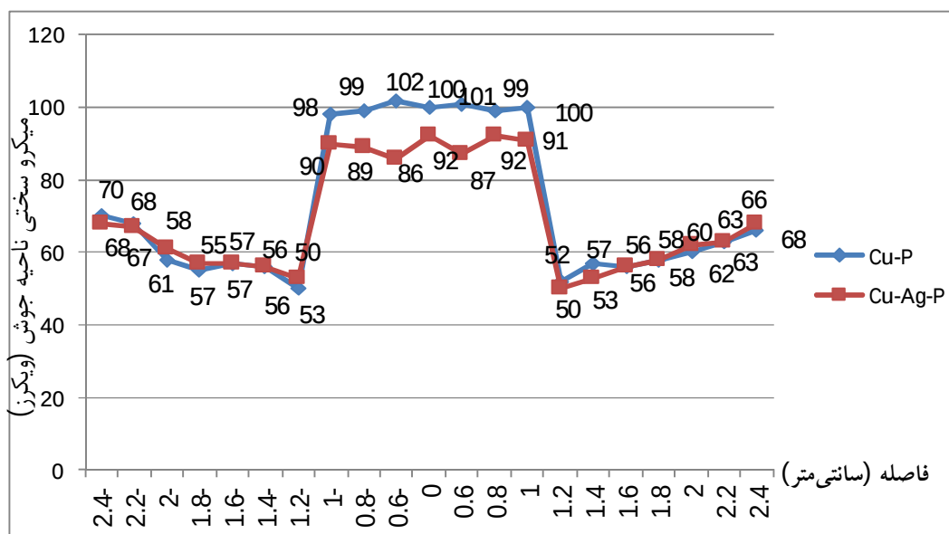
شکل 2- پروفیل سختی برای ناحیه جوش برای دو پرکننده مس - فسفر و مس - نقره - فسفر
