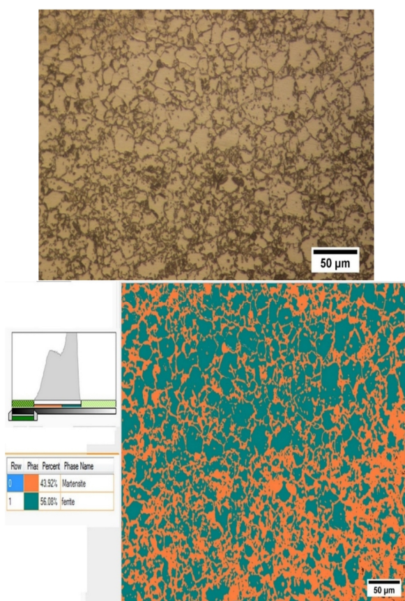
شکل 1- تصویر میکروسکوپی از فولاد پیشرفته استحکام بالا DP590 شامل مارتنزیت تمپر شده در زمینه فریت
