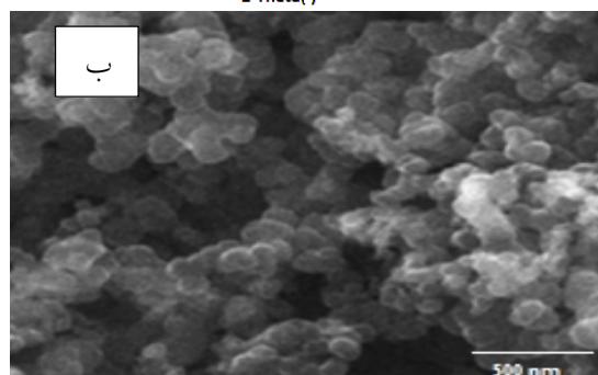
شکل 2- الف) الگوی پراش پرتو ایکس نانو ذرات ZrO_2 و ب) تصویر میکروسکوپی الکترونی روبشی از نانو ذرات ZrO_2
