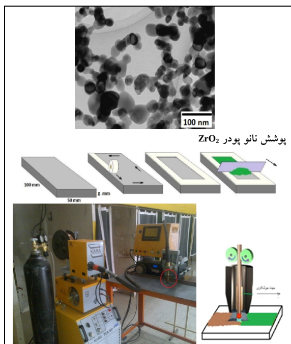
شکل 3- آماده سازی و انجام فرآیند جوشکاری نمونه ها
