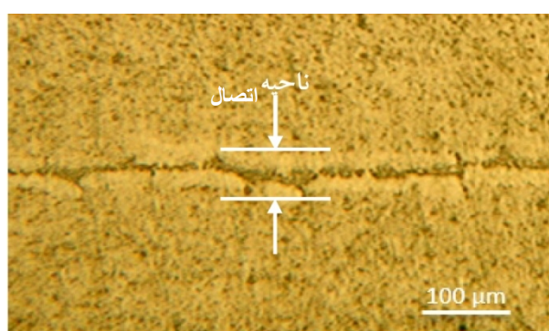
شکل 10-الف) ریزساختار ناحیه اتصال و ب) آنالیز خطی ناحیه اتصال لچیم.
