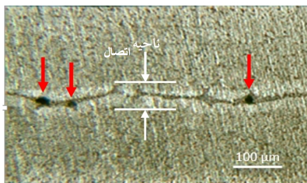
شکل 11- ریزساختار ناحیه اتصال نمونه روانساز خشک شده در دماهای، الف) 220^{\circ}\text{C} ، ب) 300^{\circ}\text{C} ، ج) 380^{\circ}\text{C} ، د) 380^{\circ}\text{C}-\text{N}_2 .
