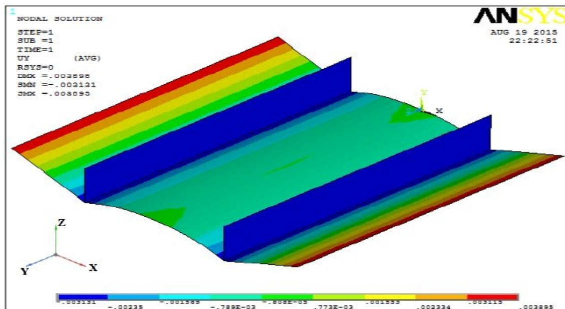
شکل ۲۰- جابجایی در راستای قائم برای حالت ((ج)) شکل-ض. کماتش در ورق
