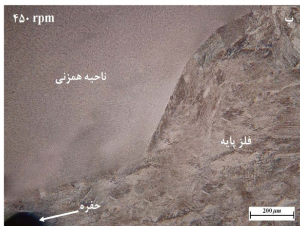
شکل 3- عیوب در مرز پایین از ناحیه همزنی در الف) 300،
