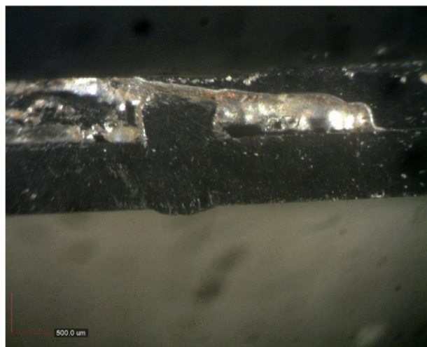
شکل 21- تصویر میکروسکوپی نوری از نمونه بهینه جوشکاری شده بعد از تست خوردگی.
