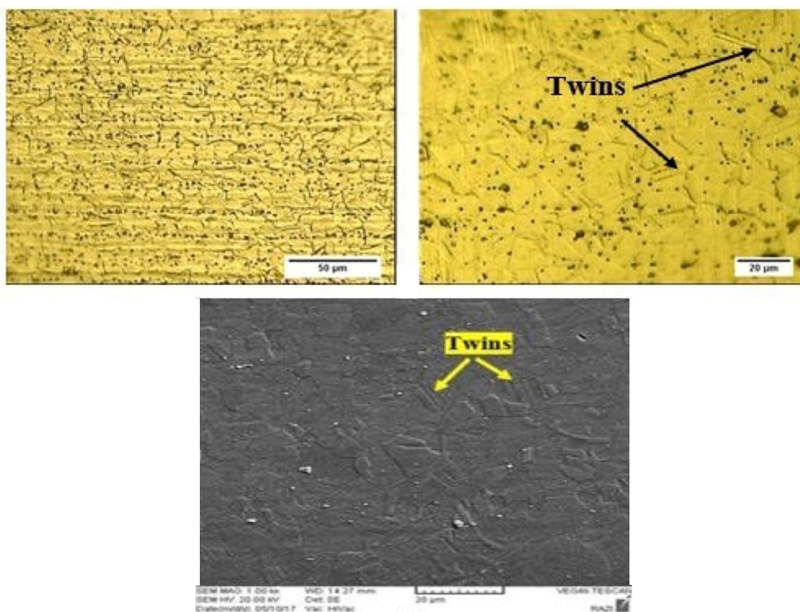
شکل 3- تصویر میکروسکوپی نوری و میکروسکوپی الکترونی روبشی مربوط به ریزساختار اینکونل 625.
