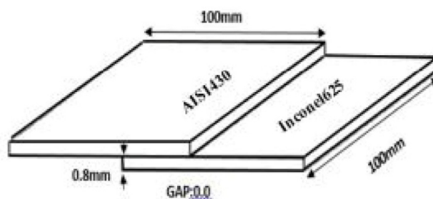
شکل 1- نمایی از طرح اتصال و نگهدارنده مورد استفاده و راه اندازی آزمایش
