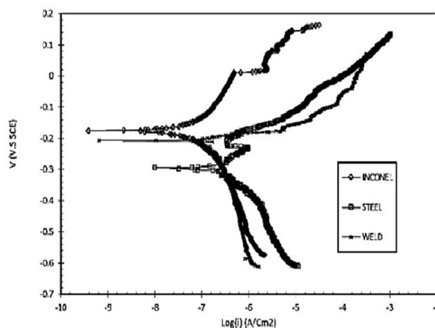
شکل 20- مقایسه نمودار پلاریزاسیون تافل نمونه های اتصال و فلزات پایه.
