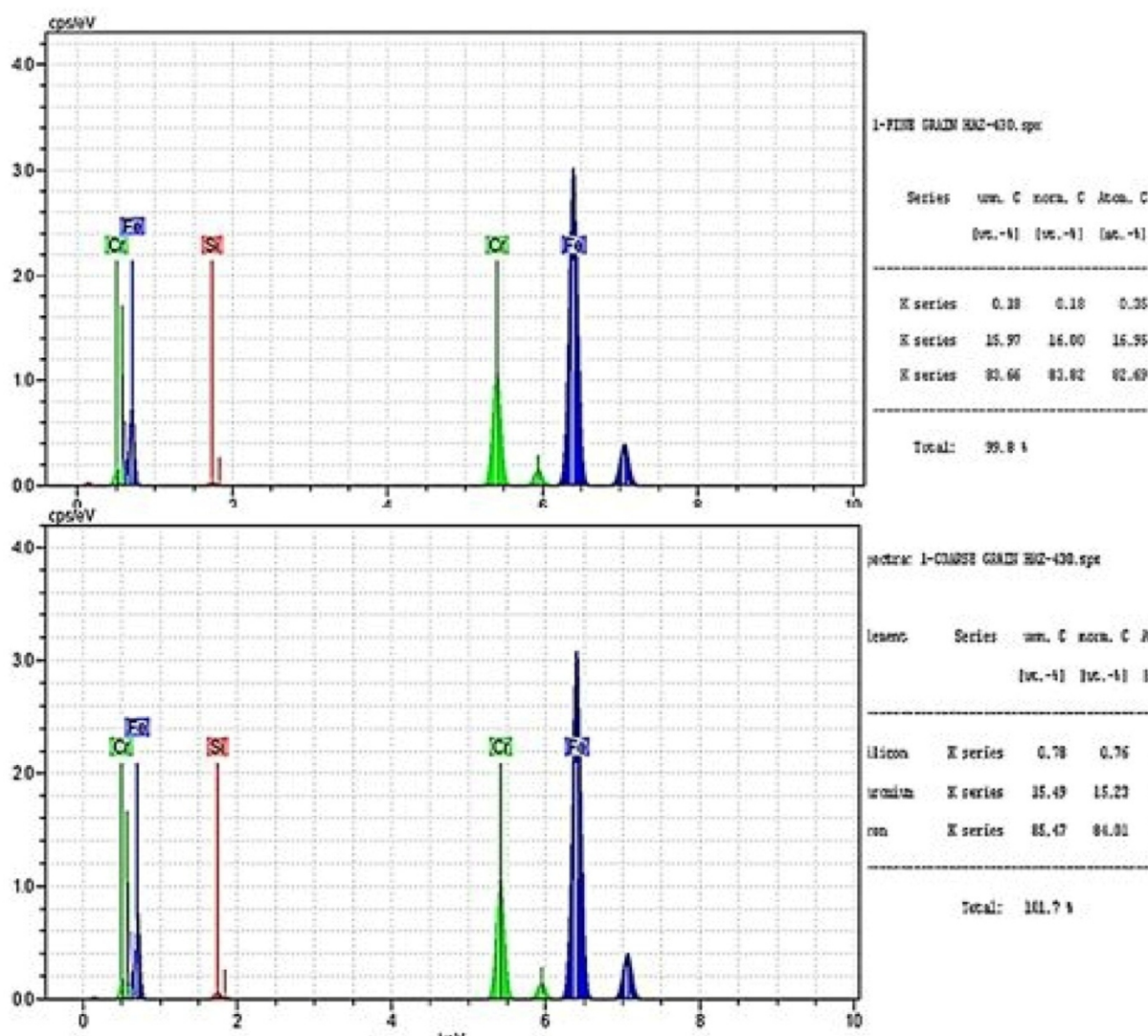
شکل 11- طیف نگاری آنالیز عنصری EDS مناطق دانه ریز و دانه درشت در منطقه HAZ فلز پایه فولاد زنگ نزن 430.
