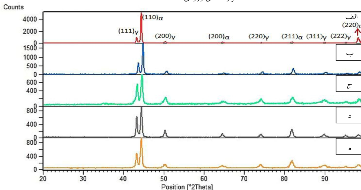
شکل ۱۱- الگوی پراش پرتوی ایکس بدست آمده برای فلز پایه و نمونه های جوشکاری شده به روش GTAW. (الف)
