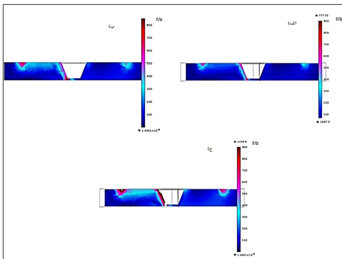
شکل ۱۳- کانتورهای توزیع نرخ کرنش در مقطع عرضی در سرعت های چرخشی مختلف. سرعت 350 RPM (الف)، سرعت 500 RPM (ب) و سرعت 700 RPM (ج)
