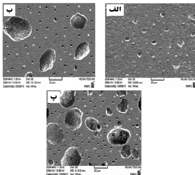
شکل ۹- تصاویر SEM از سطح خوردگی: الف) فلز پایه، ب) فلز جوش ایجاد شده با حرارت ورودی ۱۱/۲۵ kJ/mm
