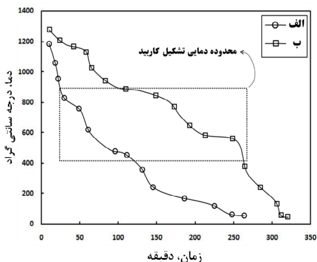
شکل ۴- نرخ سرد شدن فلز جوش اتصال جوشکاری ایجاد شده با حرارت ورودی: (الف) ۶/۷۵ kJ/mm، (ب) ۱۱/۲۵ kJ/mm
