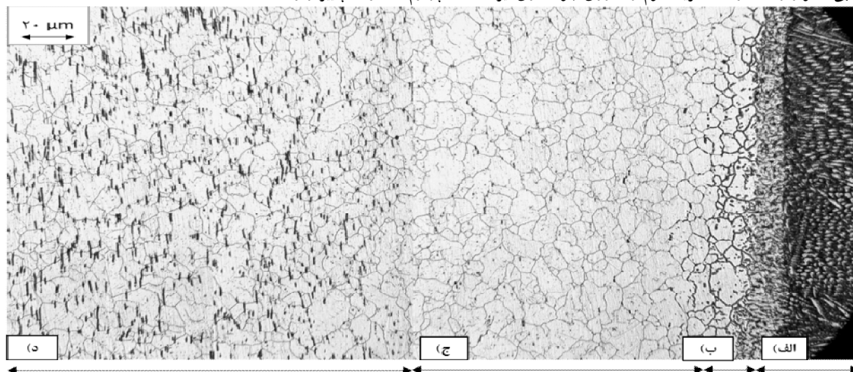
شکل ۸- ریزساختار نواحی مختلف جوش هیبریدی H1: الف) حوضچه مذاب، ب) ناحیه PMZ، ج) ناحیه HAZ و د) فلز پایه.
