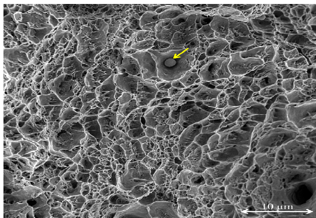
شکل ۱۱- تصویر SEM سطح مقطع شکست از فلز پایه ۴۱۳۰
